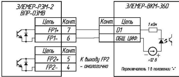
Рисунок А.10 – Схема электрическая подключений вычислителя расхода универсального «ЭЛЕМЕР-ВКМ-360» к дискретным выходам ЭЛЕМЕР-РЭМ-2 с ВПР-03МВ. R H = 1 кОм. Подключение к цепям «+FP2» и «-FP2» аналогичное
