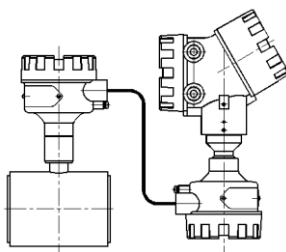
Рисунок 2.2 – Общий вид ЭЛЕМЕР-РЭМ-2-485 (раздельное исполнение)
