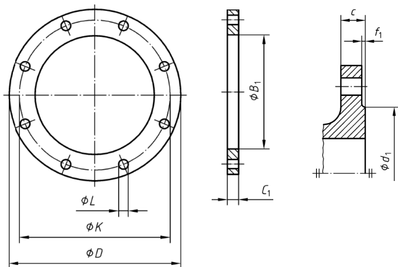
Тип фланца 01
