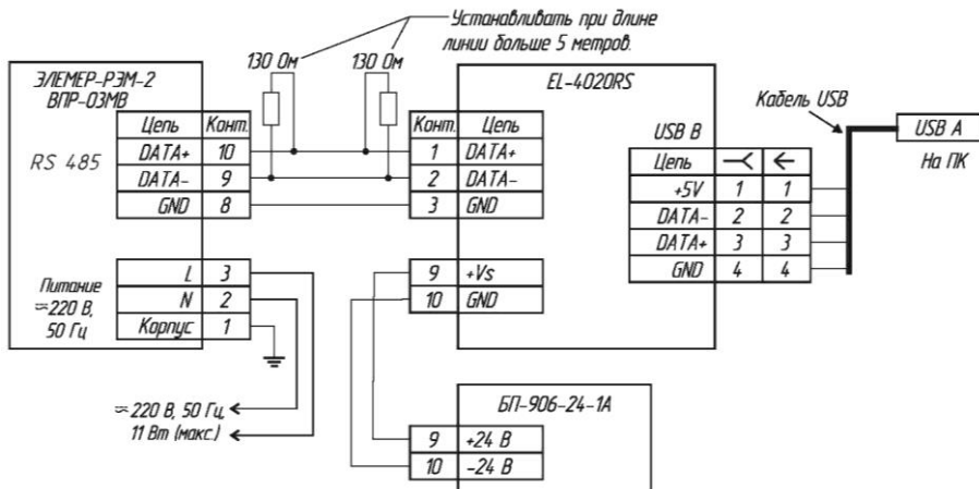
Рисунок А.18 – Схема электрическая подключений ЭЛЕМЕР-РЭМ-2 с ВГР-03МВ по протоколу обмена ModBus (источник питания 220 В)
