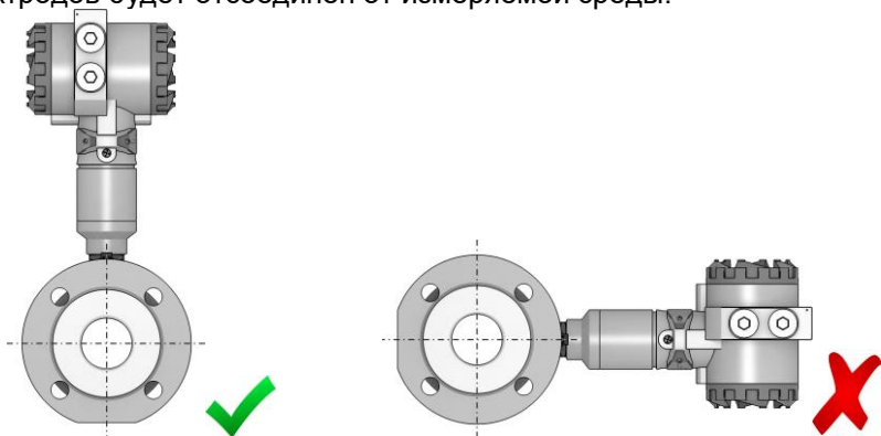
Рисунок 3.3 – Монтаж расходомера в горизонтальном трубопроводе
